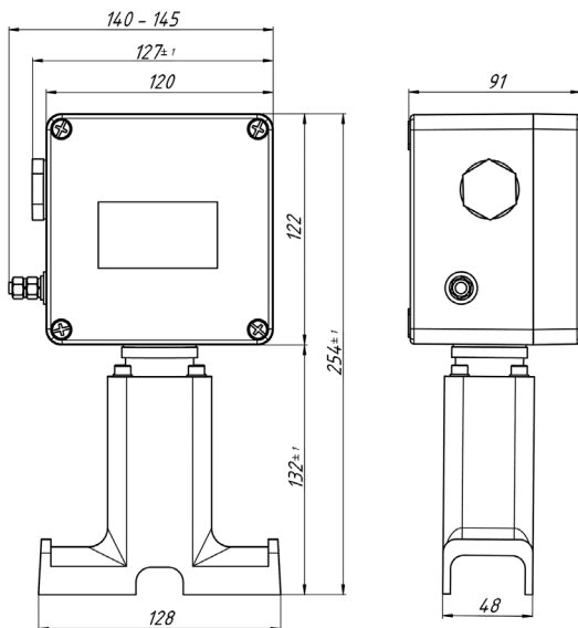
Габаритные размеры
